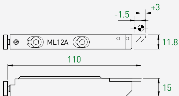
ML12A
