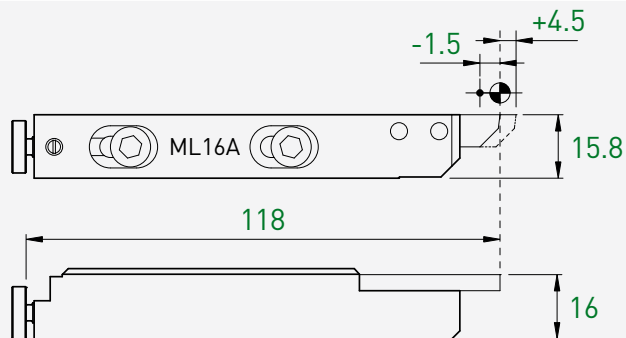
ML16A
