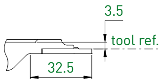
TOP-Line 731R
